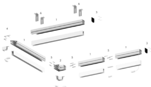
Схема сборки трековой системы SMART PROFI
