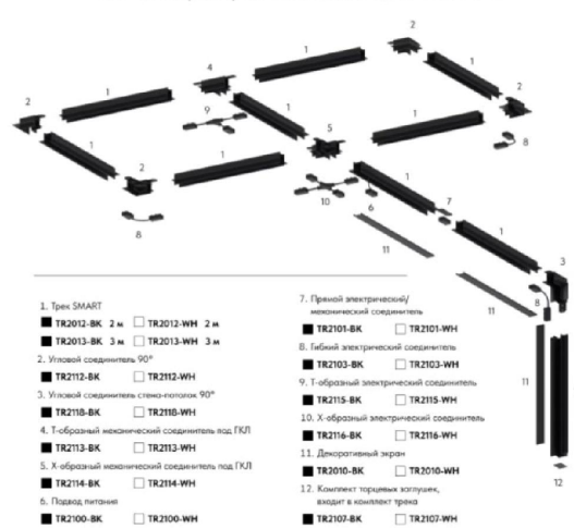
Схема сборки трековой системы SMART HIDE
