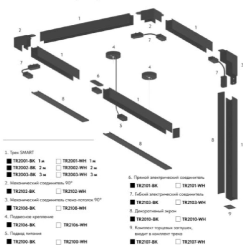
Схема сборки трековой системы SMART BASE
