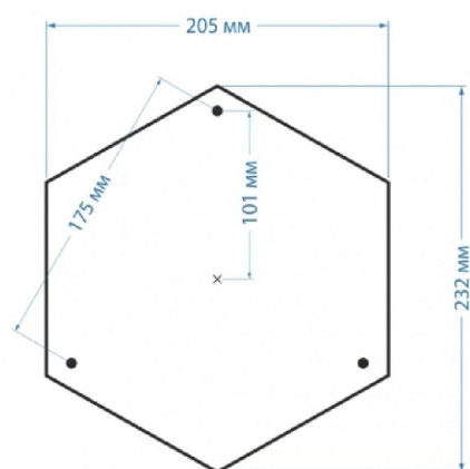
Основание светильника
